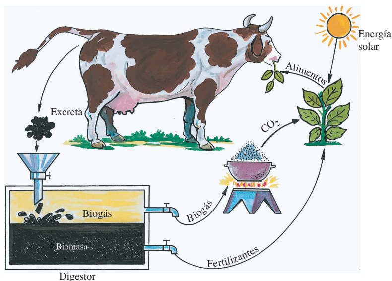
Fig. 3.19 Ciclo de la biomasa, el biogás y los deshechos en un sistema con digestor.
